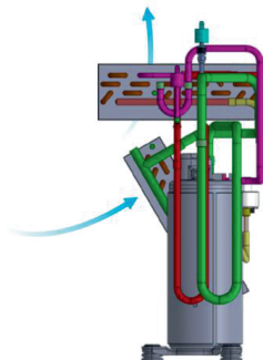
Рисунок 1 Внутренняя циркуляция хладагента в осушителе воздуха
