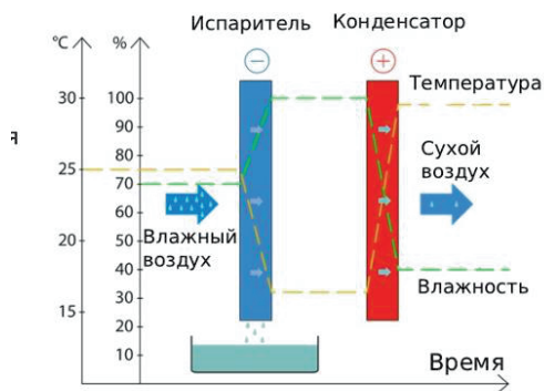
Рисунок 2 Внешняя циркуляция воздуха при осушении
