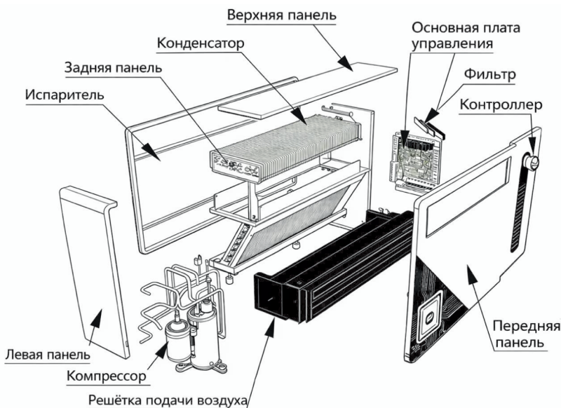
Взрыв-схема изделия
